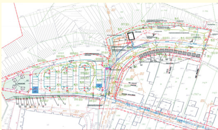
Plan przebudowy ul. Kościelnej wraz z budową parkingu oraz małej targowicy.
